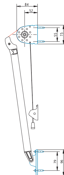
Väggmontering DA22.
