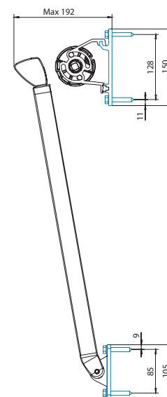
Väggmontering DA52 (mm).
